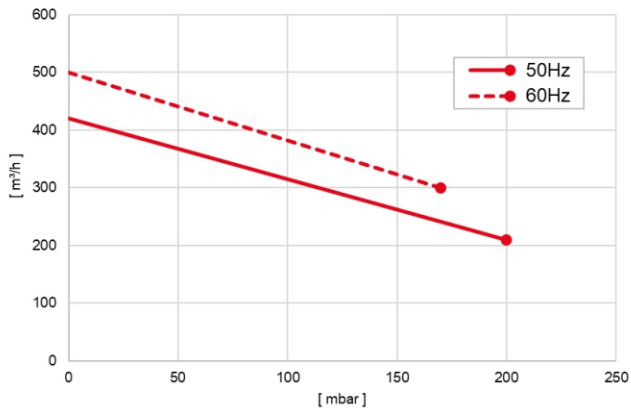
MANDATA - PRESSURE
